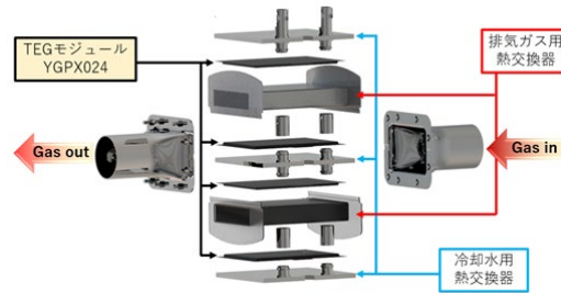
排熱発電ユニット構成
